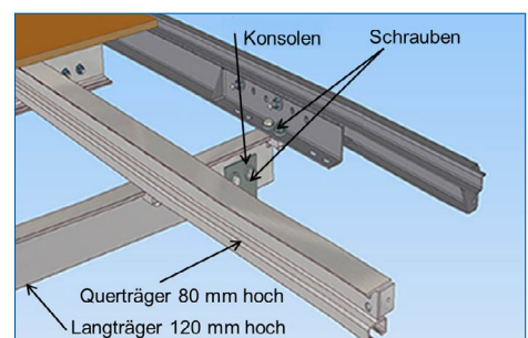
Konstruktionsprinzip
